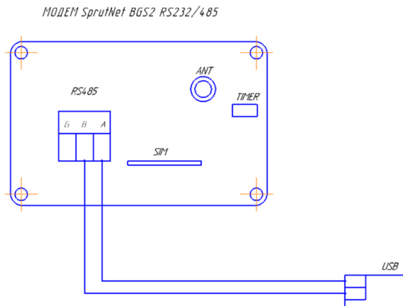
Рис.5 .Подключение модема к персональному компьютеру через адаптер USB/RS485
