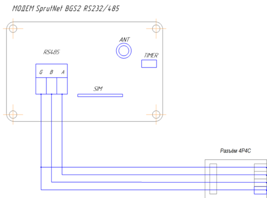
Рис.6 .Подключение к табло АЗС и в ведущую плату
