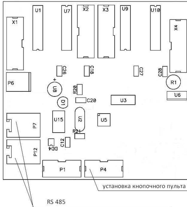
Рис.3. Ведущая плата управления
