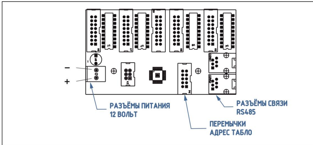
Рис.3. Ведущая плата управления
