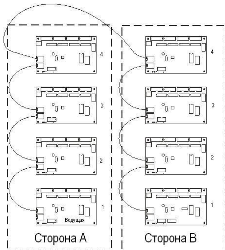
Рис.4. Схема соединения плат
